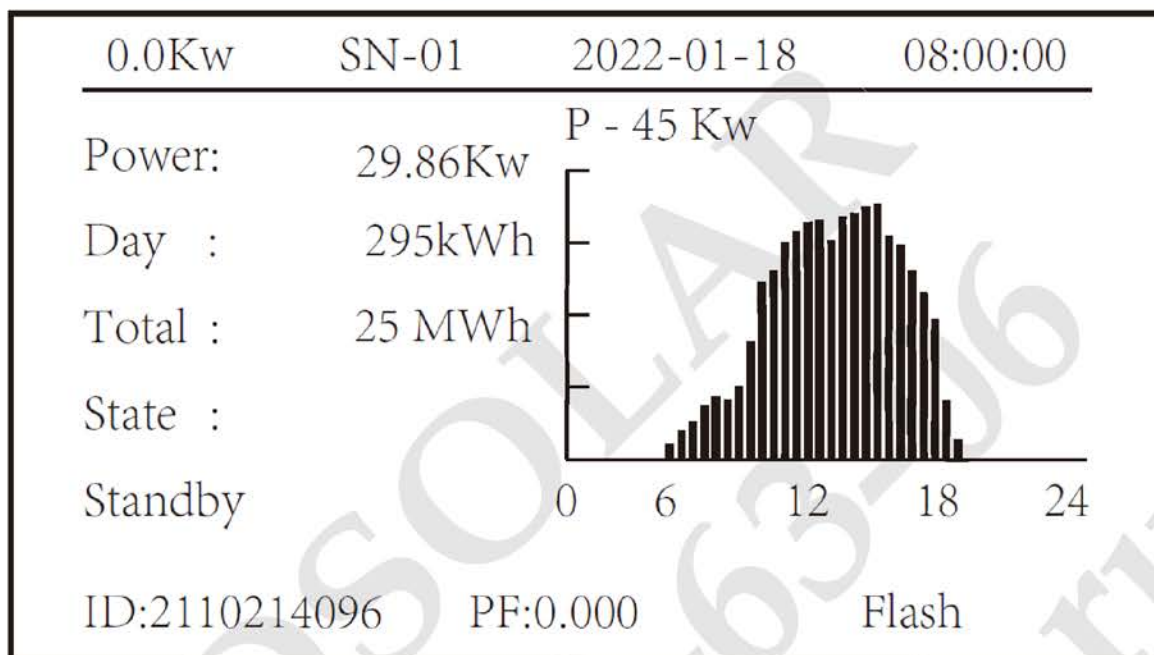
Начальный интерфейс
